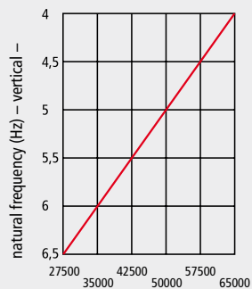
FAEBI® 430-HD load (N)
