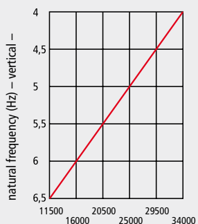
FAEBI® 300-HD load (N)
